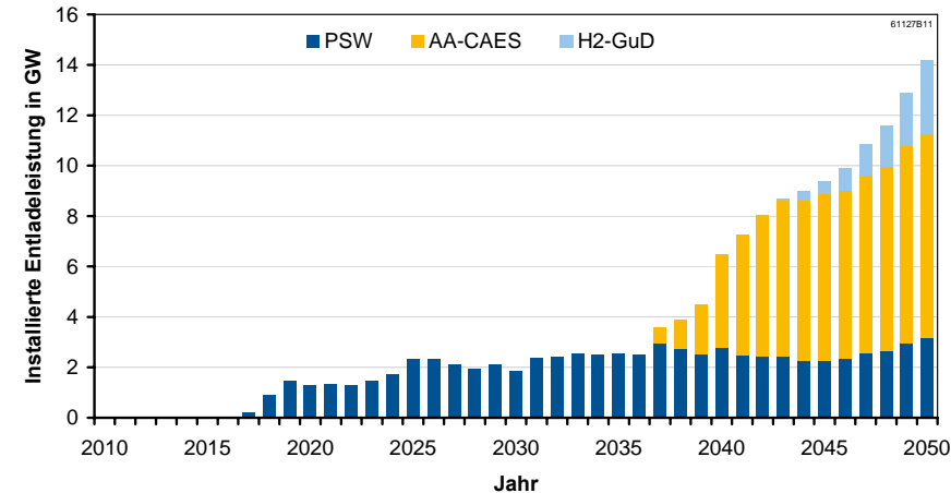
Ausbau großtechnischer Speicher in Deutschland bei 80 % regenerativer Stromerzeugung im Jahr 2050
